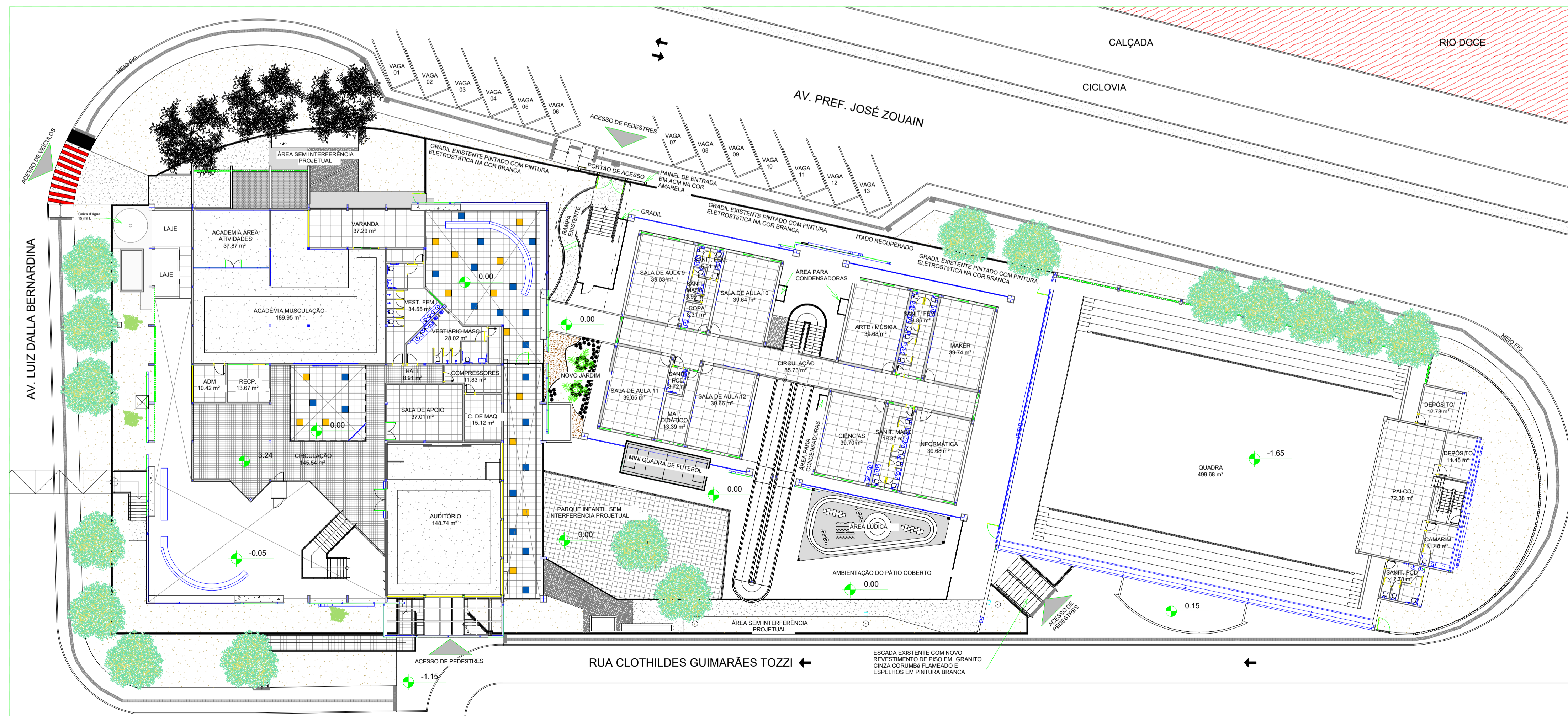
2 PLANTA GERAL - 1º PAVIMENTO 1 : 250
